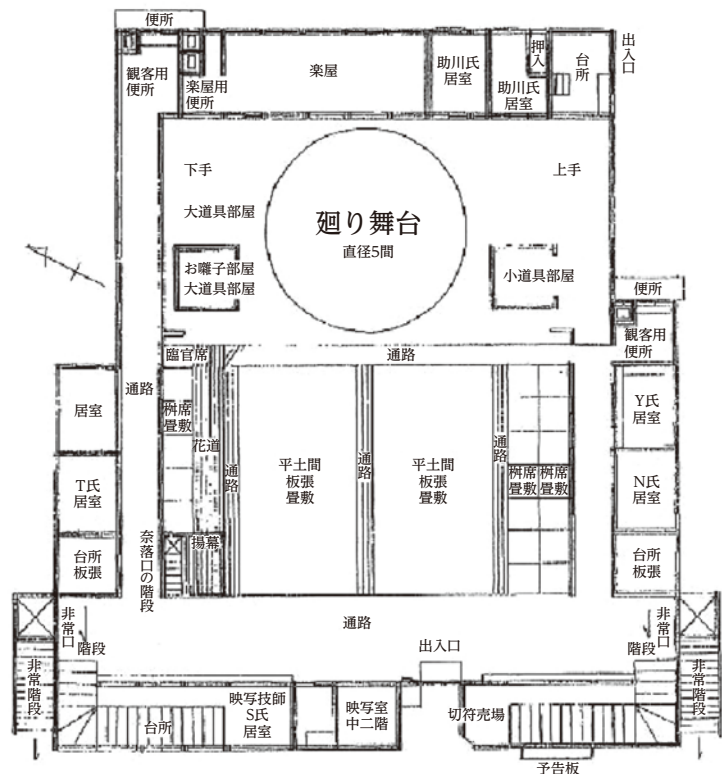
東武劇場 1階平面図 作図 故・三浦栄市
